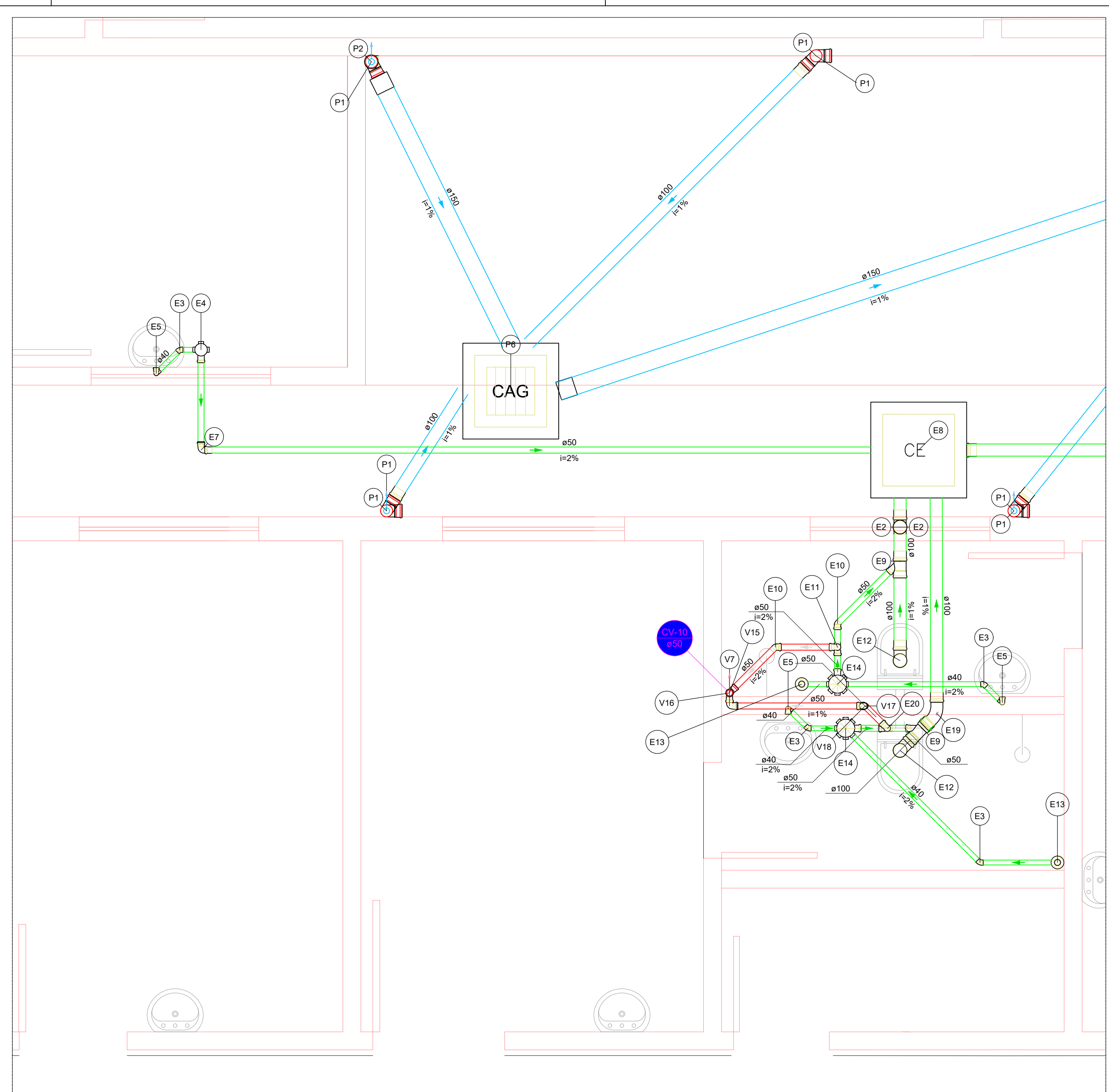
1 DETALHE S14 1:25
