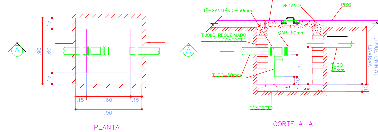
CAIXA DE GORDURA 60x60cm ESCALA 1:25
