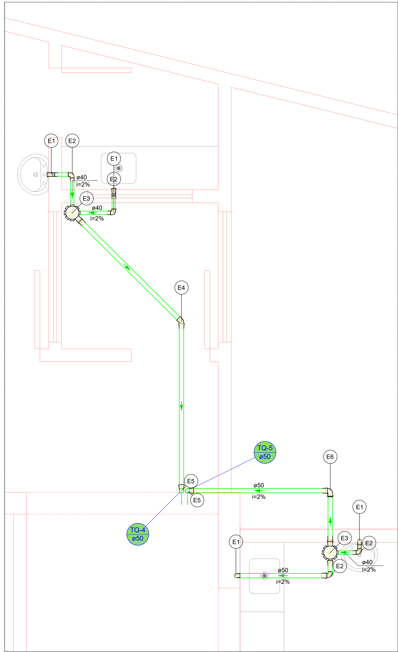
2 DETALHE S6 1:25
