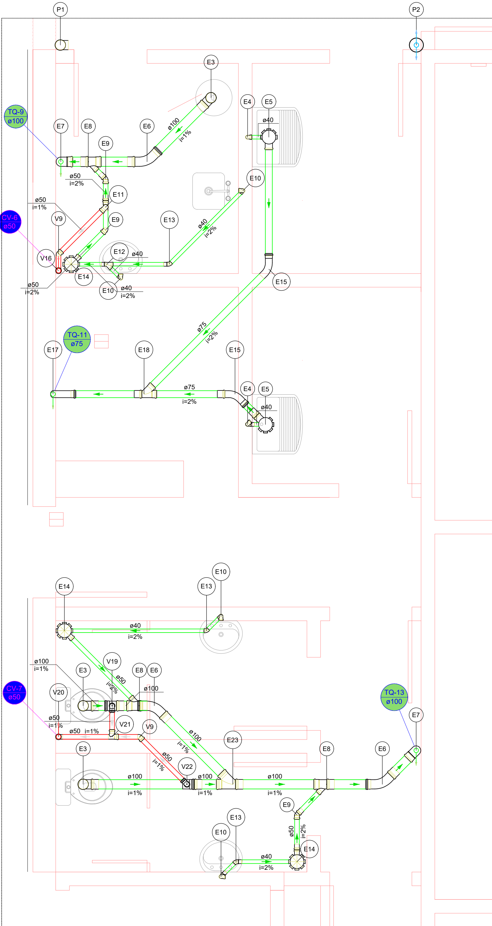
1 DETALHE S11
