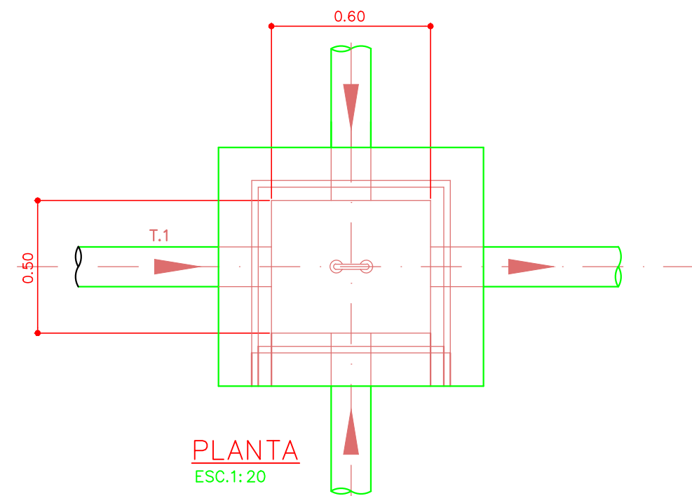
DETALHE CAIXA DE INSPEÇÃO ESC.1:20
