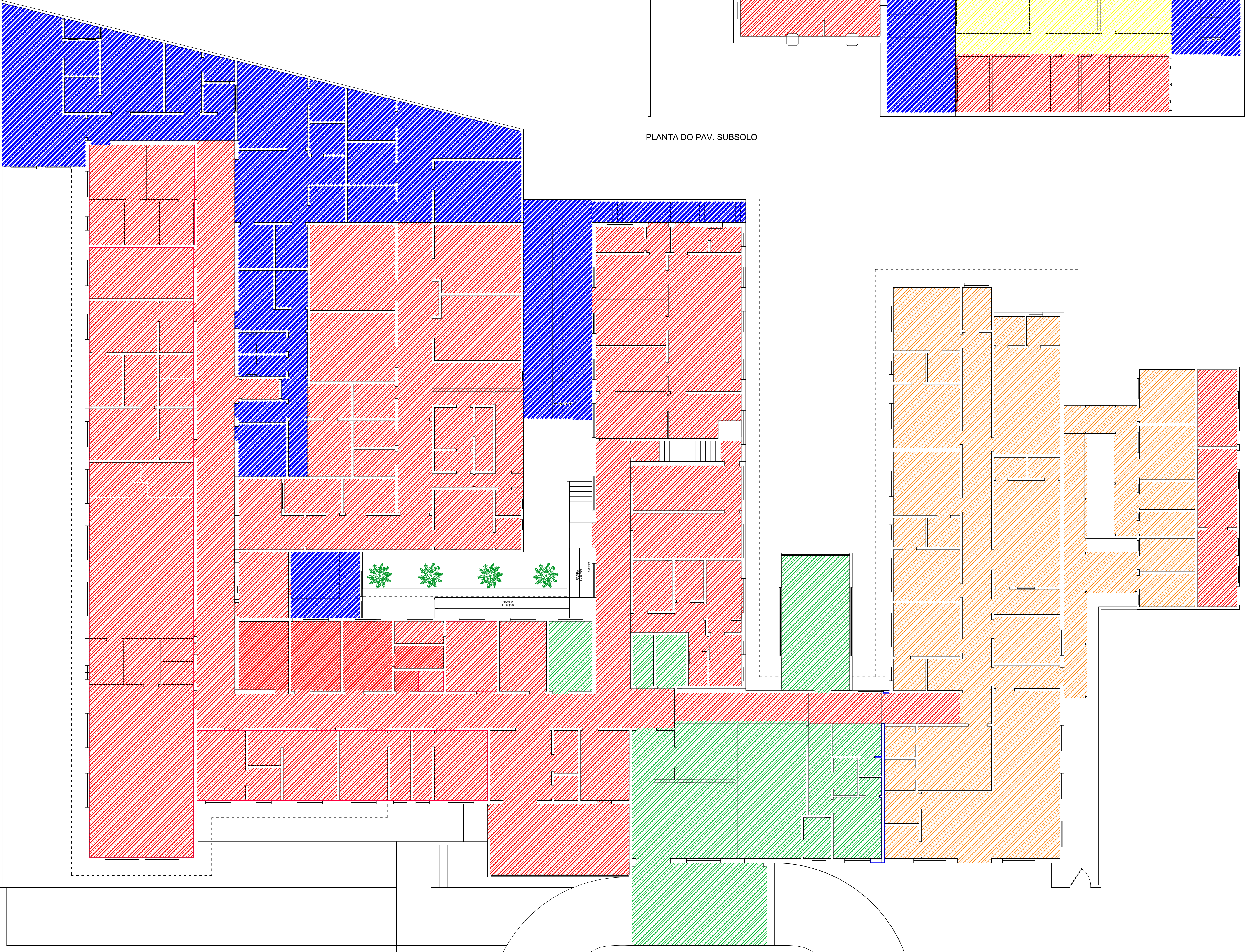
PLANTA DO PAV. TÉRREO
