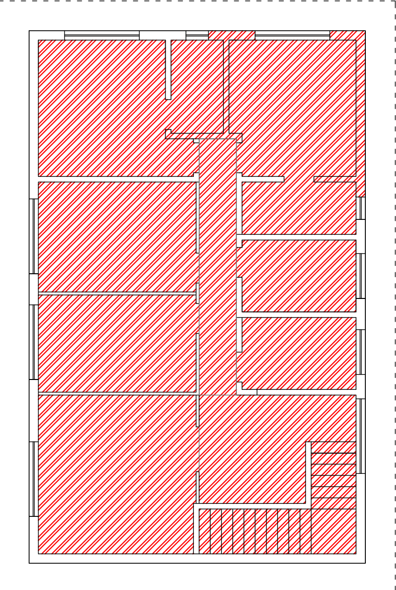
PLANTA DO PAV. SUPERIOR
